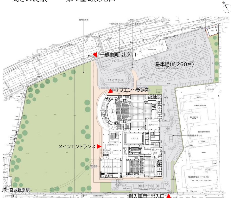
配置図
